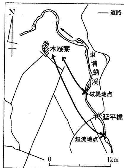
図10 東埔蚋溪での越水・破堤氾濫
