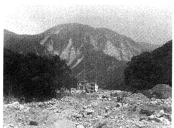
写真3 南投県水里郷上安村郡坑で発生した土石流によって被害を受けた家屋（背後の山には多数の斜面崩壊が見られる）
