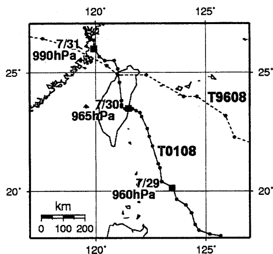
図1 台風0108号の経路(日付表記位置(■)は各日0時の中心位置。気圧は0時の中心気圧)
