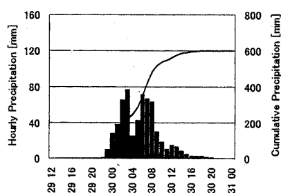
図9 主要観測所の1時間降水量及び積算降水量（光復観測所の7月30日04時以降は欠測の模様）
