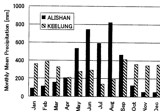
図 4 阿里山 (Alishan) と基隆 (Keelung) の月別降水量平年値 (1961～1990 年)
