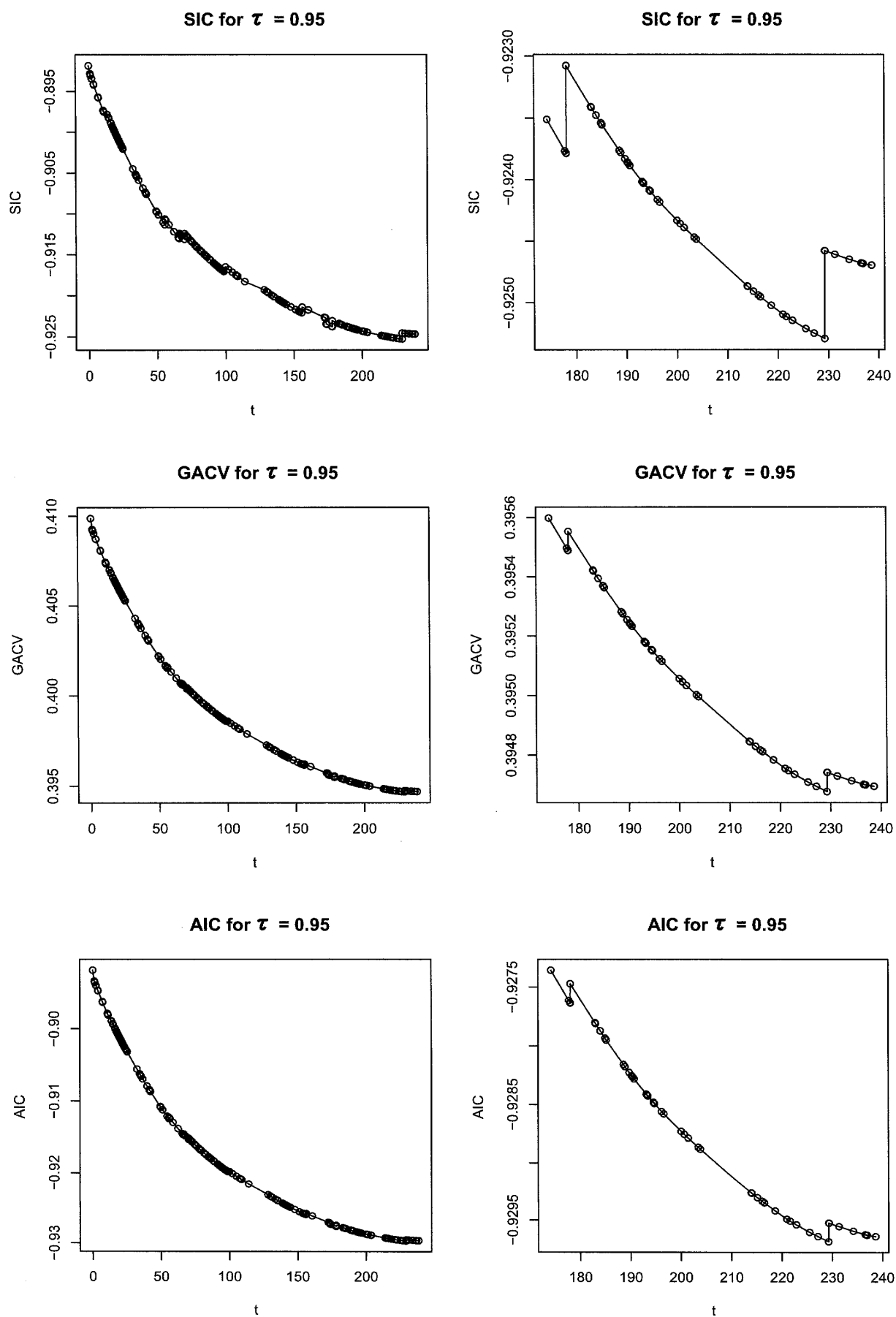
図 15 Lasso 分位点回帰 ( \tau=0.95 ) におけるモデル選択規準の値：上段：SIC，中段：GACV，下段：AIC
