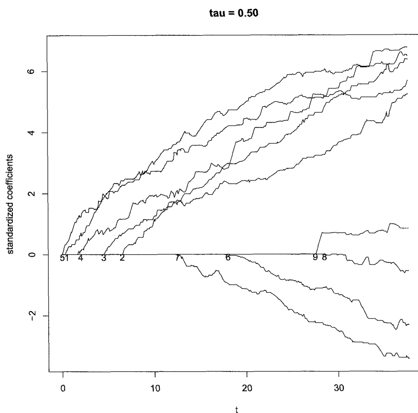
図 12 Lasso 分位点回帰の結果 ( \tau=0.50 )
