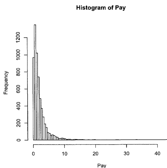
図1 クレーム額のヒストグラム
