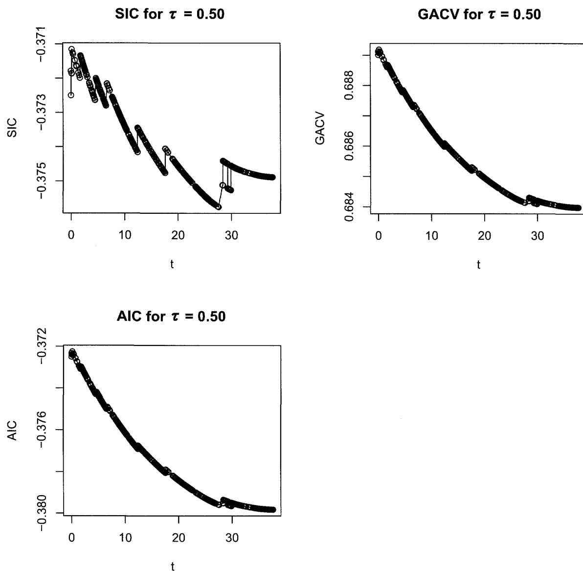
図 14 Lasso 分位点回帰 ( \tau=0.50 ) におけるモデル選択規準の値：上段左：SIC，上段右：GACV，下段：AIC
