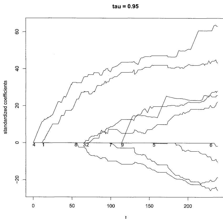
図13 Lasso 分位点回帰の結果 ( \tau=0.95 )
