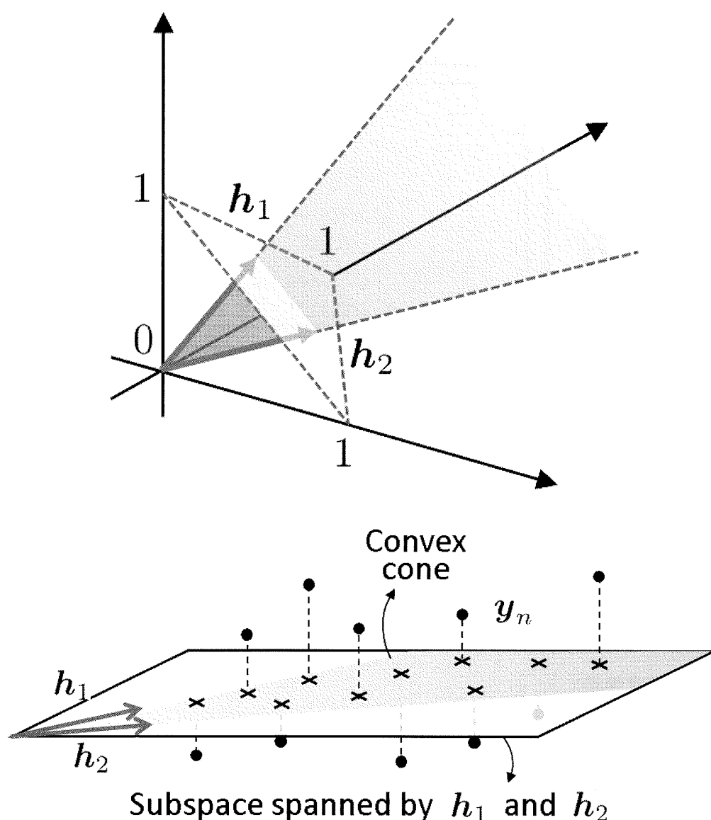
図2 NMFの幾何学的イメージ.
