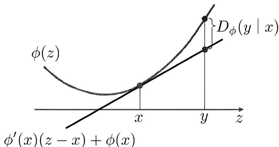
図6 Bregman ダイバージェンス.
