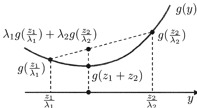
図5 Jensen の不等式 ( I = 2 の場合).
