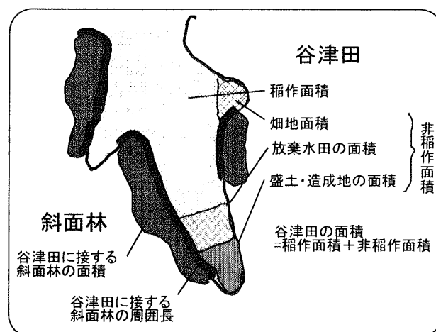
図-1 谷津環境における土地環境の模式図
