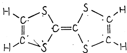
TTF
