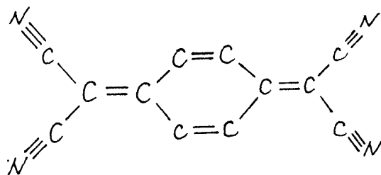
TCNQ
