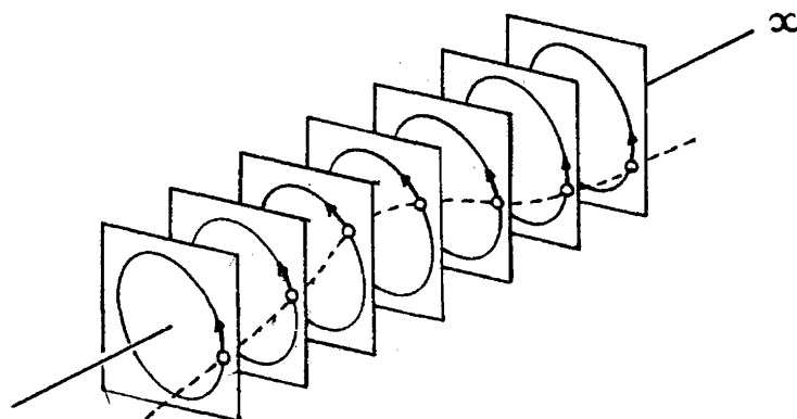
図1 空間座標 x 上に分布したリミットサイクル。位相の空間変化がゆるやかであれば、状態点はほぼリミットサイクル軌道にある。
