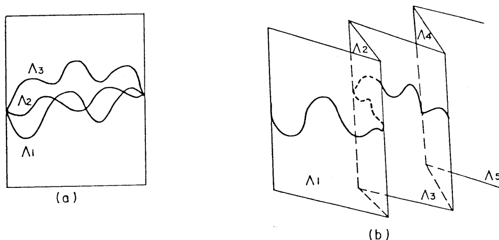
図 1. (a) “ミミズのトンネル”の標本経路。(b) A_{2n} 上では、漸化式の \tilde{P}_t^{\alpha} の変換 ( \tilde{P}_t^{\pm} \rightarrow \tilde{P}_t^{\mp} ) を行うと(a)の標本経路は 1 本の長いトンネルになる。
