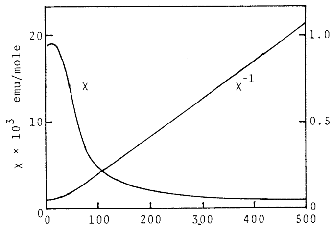
図3 磁化率( \parallel c ) 文献(5)
