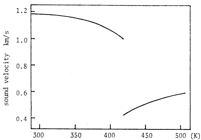
図11 音速 文献(8)
