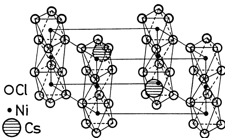
図1 \text{CsNiCl}_3 型の結晶構造
