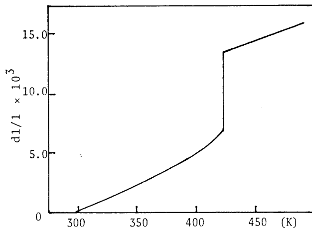
図8 熱膨張( c 軸) 文献(6)
