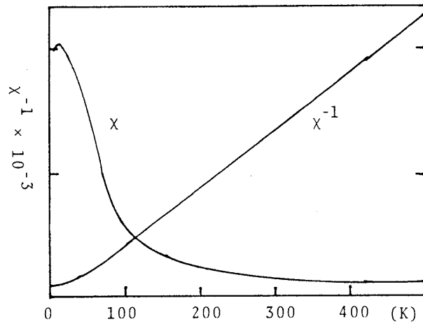
図4 磁化率( \perp c ) 文献(5)
