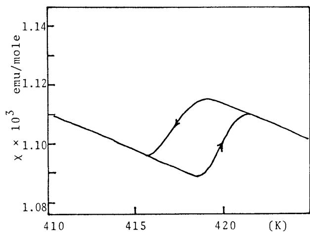
図5 磁化率( \parallel c ) 文献(5)
