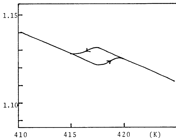
図6 磁化率( \perp c ) 文献(5)
