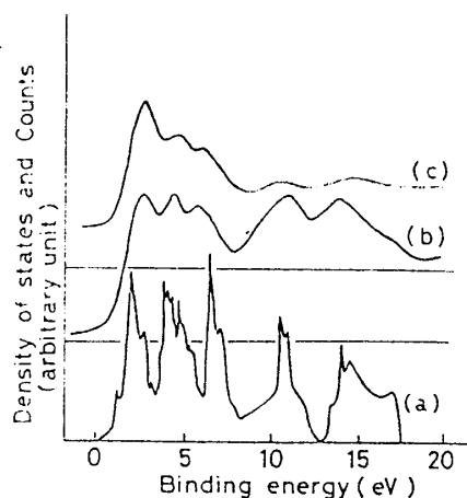
★5図 a) DOS, b) XPS, c) UPS.
