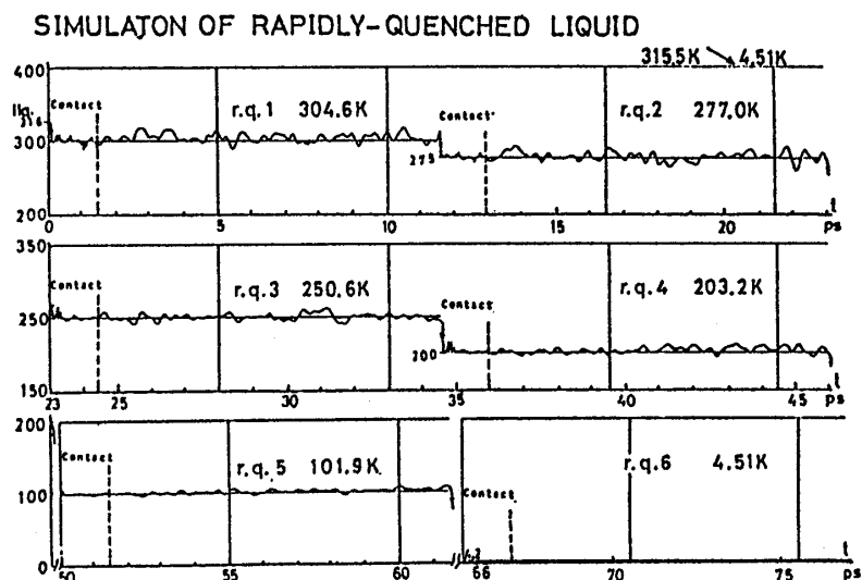
図5. 熱源接触法による液体金属超急冷法のシミュレーション：温度 (K, E(t) ) の時間的変動。 各中間温度では定常状態にある。
