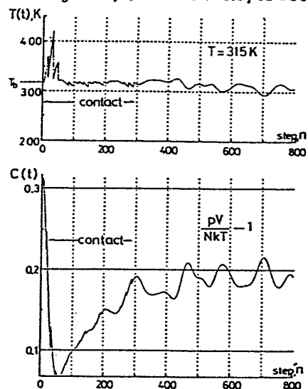
図 2. 「熱源接触法」による初期条件の補正の例 (横軸は 800 ステップまでを拡大して示す)。
