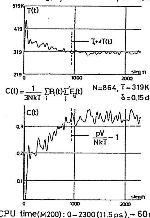
図1. 初期条件の不備による全運動エネルギー K.E.(t) 、ビリアル C(t) の変動
