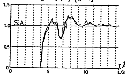
図 8. 3体分布関数 g^{(3)}(r, s, t) の計算例：正三角形相関 g^{(3)}(r, r, r) (上) と superposition approximation との比較(下)：下図の細かい凹凸の大部分は統計誤差による。
