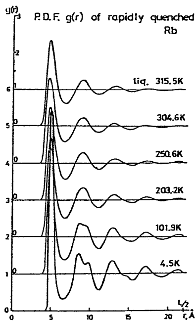
図 7. (a) 急冷過程における g(r) の変化
