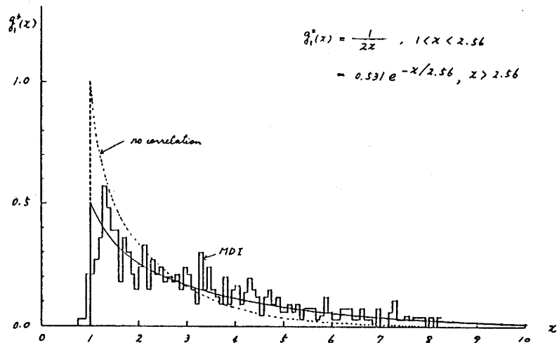
第2図 1体分布のスケーリング関数
