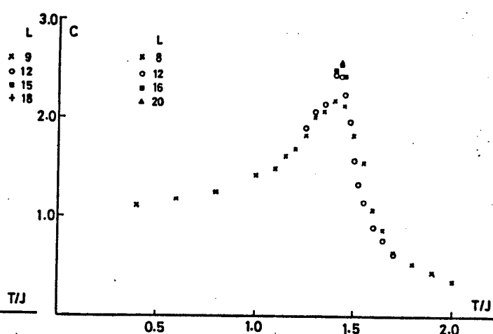
図3 単純立方格子上の強磁性的古典ハイゼンベルクモデルの比熱のサイズ、温度依存性。
