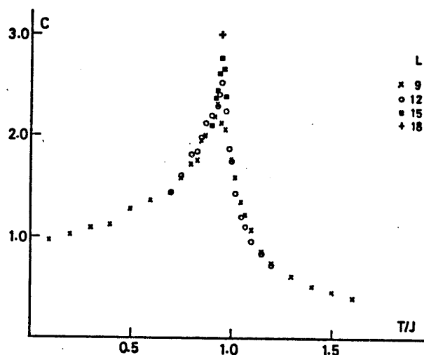
図2 比熱のサイズ、温度依存性
