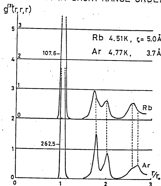
図 4. r. q. 状態での g^{(3)}(r, r, r) の相似性
