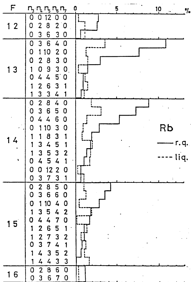
図 7. Index n_3 \sim n_7 による分類
