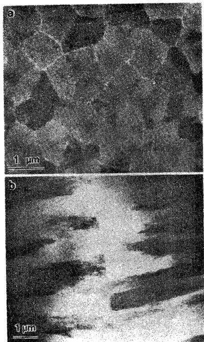
図1 急冷Al-Mn合金の透過電子顕微鏡像 (a) Al_{86}Mn_{14} (b) Al_{80}Mn_{20}
