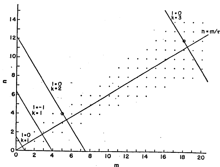
図7 式(2), (3)の解を探すための m, n 平面。丸を付けた点が解である。
