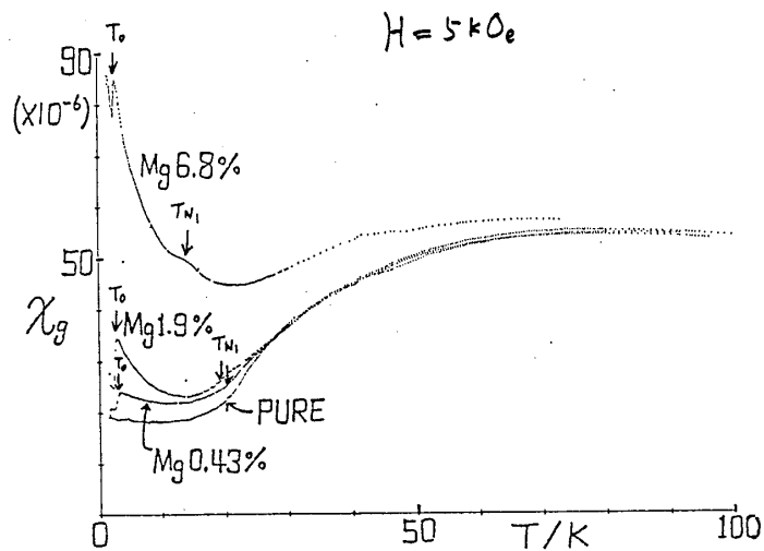
図14 \text{CsCo}_{1-x}\text{Mg}_x\text{Cl}_3 の磁化率
