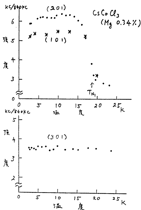
図13 \text{CsCo}_{0.9966}\text{Mg}_{0.0034} の中性子散乱の積分強度
