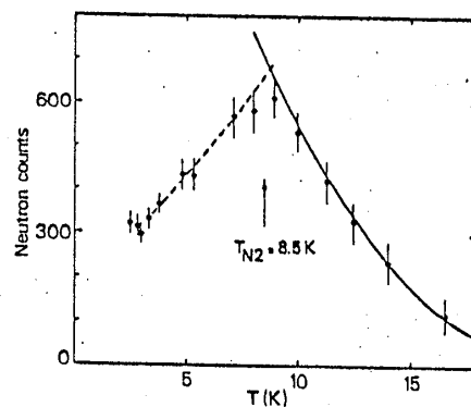
図11 \text{CsCoCl}_3 における (0.9 0.9 1) 面からの中性子磁気反射
