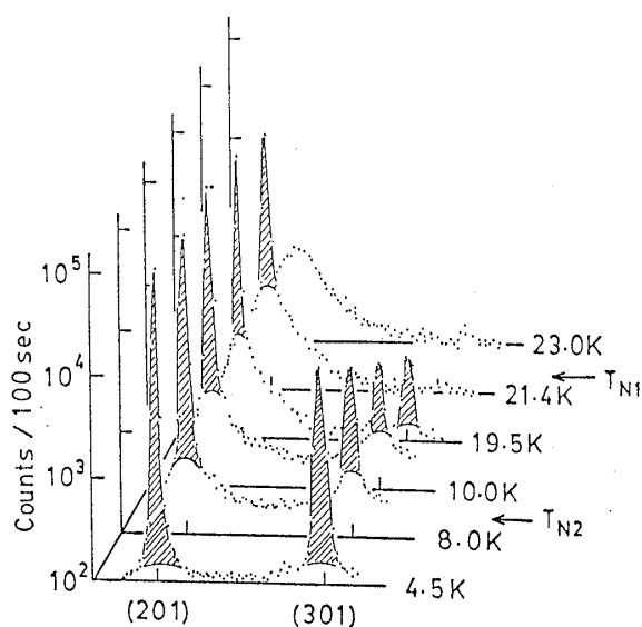
図7 \text{CsCoCl}_3 の中性子の (h01) 反射
