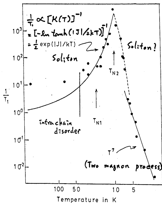
図10 \text{CsCoCl}_3 中の ^{133}\text{Cs} の NMR の T_1
