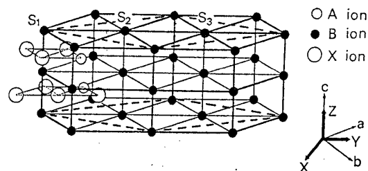
図1 CsNiCl 3 構造における磁気格子
