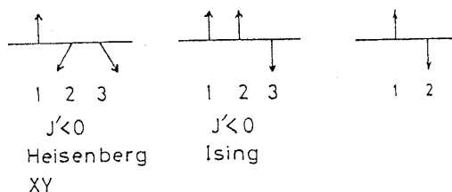
図2 古典スピンの三角格子の基底状態
