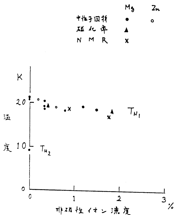
図12 \text{CsCo}_{1-x}\text{M}_x\text{Cl}_3 の転移温度
