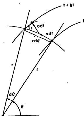
Fig.5 Cowie&Rybicki(C&R)のGalacto-Detonation Waveモデル。波面の伝搬はHuygensの原理と銀河円盤の回転とで決まる。
