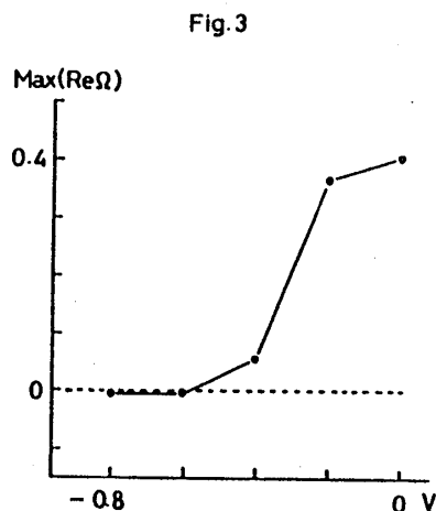
Fig.3 線形安定性解析の固有値。 m=2, Q=0.5, k=0.5 。 V<0 ほど 安定化している。
