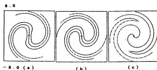
Fig.1 剛体回転するスパイラル解の例。 m=1, Q=1.0, k=0.8, V=0.0 (a), -0.5 (b), -3.0 (c)。
