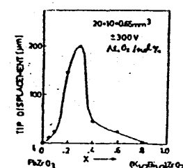
図3 PZの組成による変位量の変化
