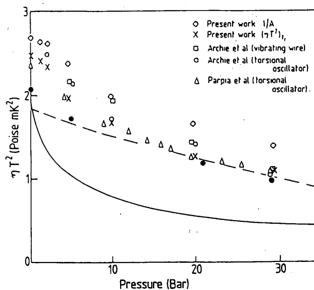
図2 T \rightarrow 0 での \eta T^2 の値 ( 1/A ) の圧力依存性のグラフ (Carless ら[2] による。)
