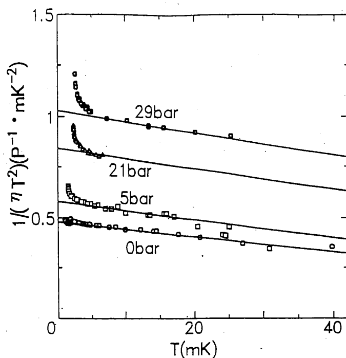
図1 1/\eta T^2 の温度依存性のグラフ
