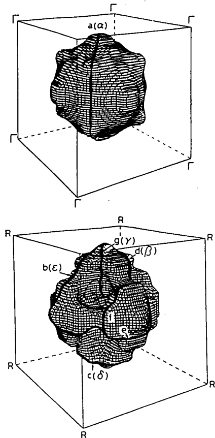
図 4: \text{CeSn}_3 のホール面と電子面
