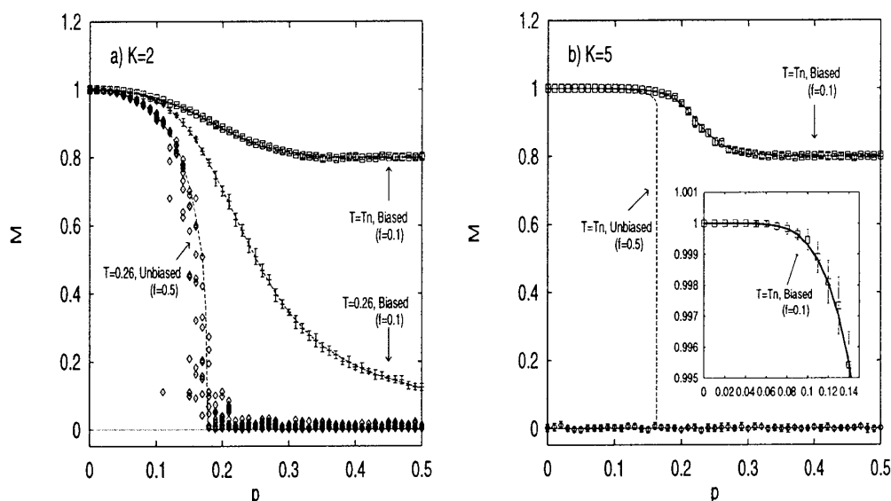
図 2: TAP 方程式を用いた復号化の実験結果。a) K = 2 、b) K = 5 とともに N = 10000 、 M = 20000 ( R = N/M = 1/2 ) の系に関して TAP 方程式を事前知識 (符号の偏り) を反映させた初期条件からそれぞれ 30 回反復させた解を用いて復号化した。マーカーは 10 回の実験での平均 (誤差棒はそれより小さい)、曲線はレプリカ法 (RS 解) による予想である。
