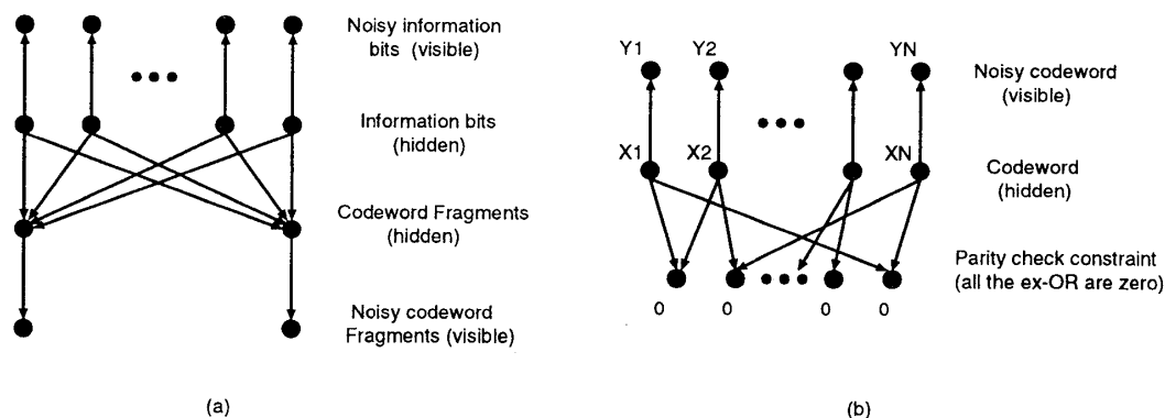
図 4: Bayesian ネットワーク (a) Turbo 符号, (b) 低密度パリティ検査符号
