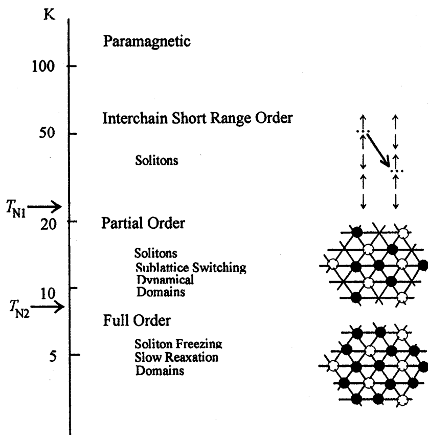
図4 \text{CsCoCl}_3 の秩序化過程。一つのc面で見て秩序化したupスピンを黒丸、downスピンを白丸で表してある。
