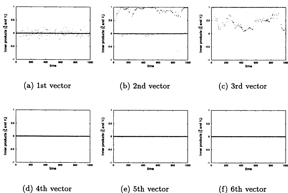
図 4: 正規化されたリアプノフベクトルと軌道の進行方向 \tilde{\xi}(t) との内積の時間変化。 E = 0.04 . 濃い直線が幾何学的方法の結果で、薄い曲線が従来の方法の結果。従来の方法では第 1, 2 リアプノフベクトルが \tilde{\xi} との直交性を保てず、第 3 リアプノフベクトルが \tilde{\xi} の方向からずれてしまうことがわかる。直交性を保てないことがわかる。(d),(e),(f) では薄い直線は濃い直線の陰に隠れてしまっている。
