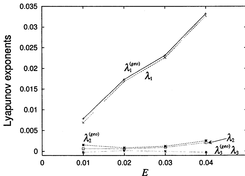
図 3: リアプノフ数のエネルギー依存性。エネルギーによらず、従来の方法と幾何学的方法とで得られたリアプノフ数は一致する。
