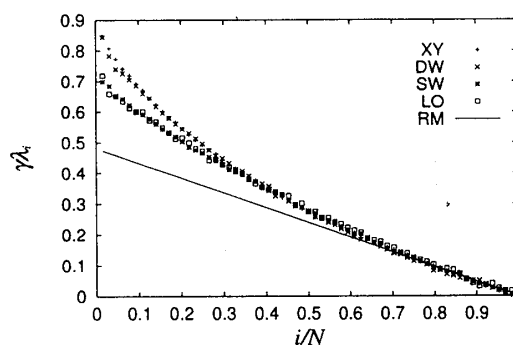
図 1: カオスが Stochastic ほど強くはない系におけるリアプノフスペクトルの普遍性。自由度 N = 4^3 = 64 。領域 i/N > 0.4 では系によらない同じ形が得られる。直線は、発達したカオス系で得られる直線スペクトルを示している。
