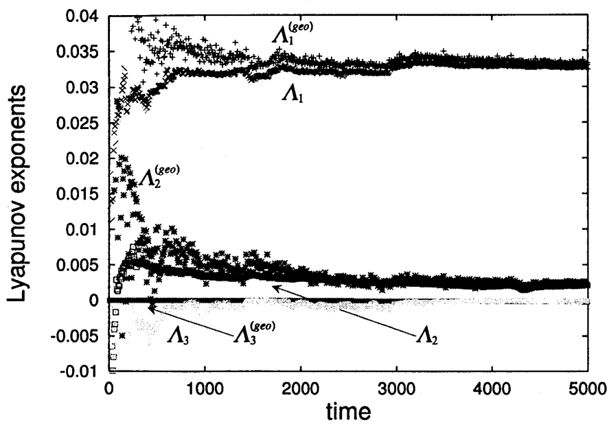
図 2: リアプノフ数の収束性。 E = 0.04 . 従来の方法と幾何学的方法を用いたリアプノフ数は同じ値に収束する。
