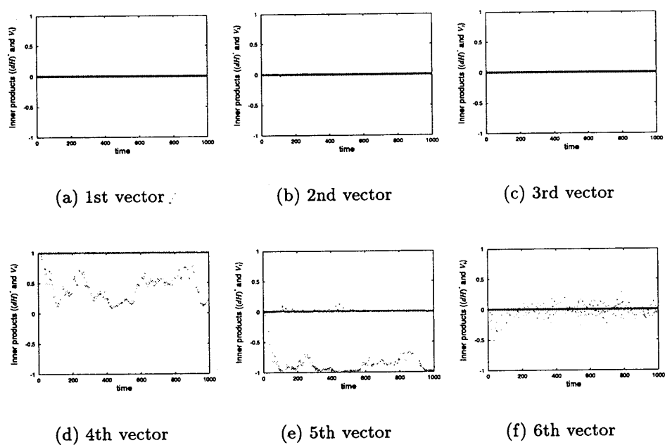
図 5: 正規化されたリアプノフベクトルとハミルトニアン勾配方向 (dH^{(\text{geo})})^*(t) との内積の時間変化。 E = 0.04 。 濃い直線が幾何学的方法の結果で、薄い曲線が従来の方法の結果。従来では第 5, 6 リアプノフベクトルが (dH^{(\text{geo})})^*(t) との直交性を保てず、第 4 リアプノフベクトルが (dH^{(\text{geo})})^*(t) の方向からずれてしまうことがわかる。(a),(b),(c) では薄い直線は濃い直線の陰に隠れてしまっている。
