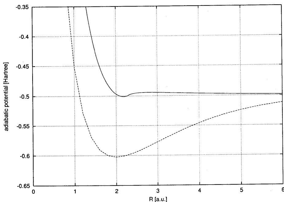
図 3: 構成条件を変更して不連続性を解消した断熱ポテンシャル (実線)。 C = C' = 0.5 。この断熱ポテンシャルは EBK 量子化したとき電子基底状態となる。破線は量子力学で得られる電子基底状態 1s\sigma_g 。2つの断熱ポテンシャルが大きく異なることがわかる。
