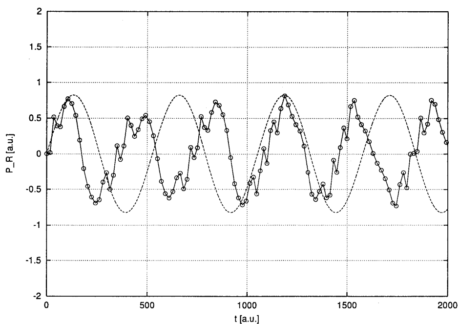
図 5: Poincaré 写像によって得られる運動量 P_R の時系列 (白丸)。図 1 と同じ軌道を元になっている。破線は断熱ポテンシャルから予想される時間発展。
