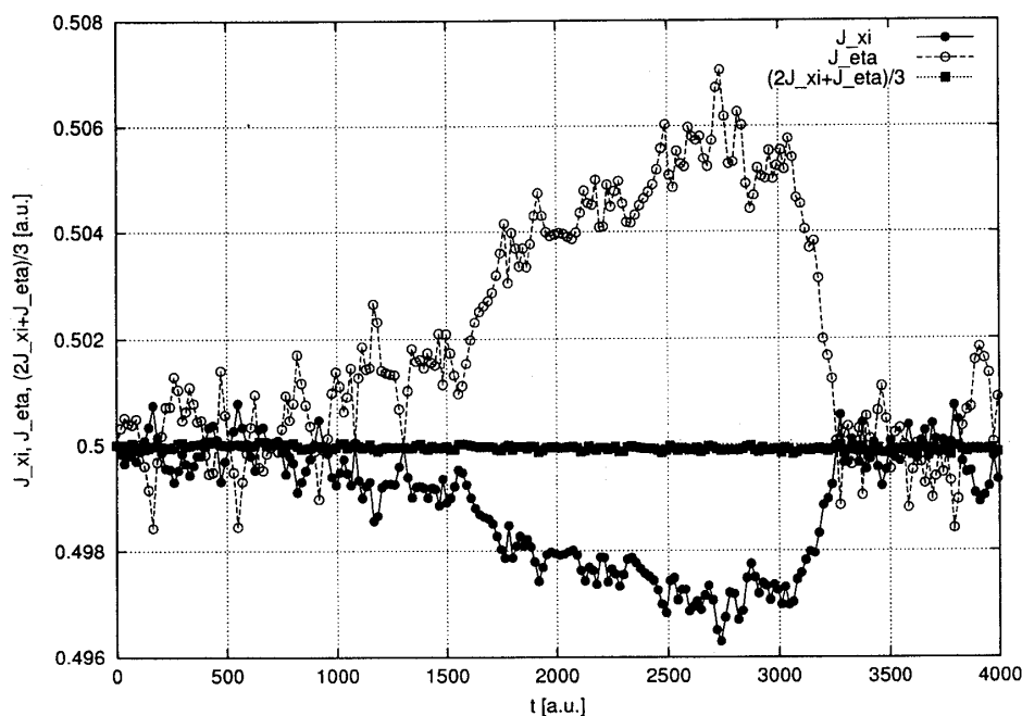
図6: Poincaré 写像によって得られる J_\xi, J_\eta, (2J_\xi + J_\eta)/3 の時系列。それぞれ、黒丸が J_\xi 、白丸が J_\eta 、黒四角が (2J_\xi + J_\eta)/3 の時系列を表す。図1と同じ軌道を元にしていて、 J_\xi, J_\eta, (2J_\xi + J_\eta)/3 の初期値はともに0.5である。
