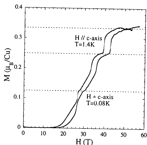
図8 磁化曲線 13)
