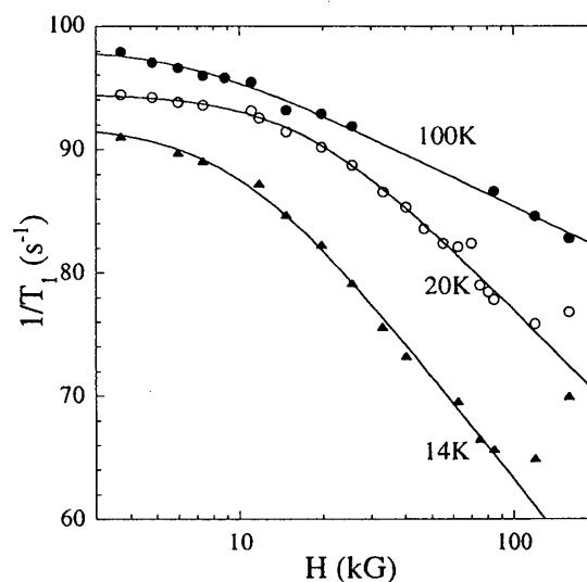
図5 1/T_1 の磁場依存性
