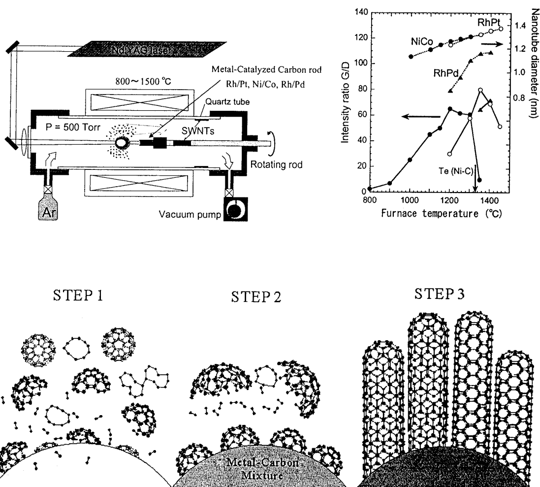
図1 左上 レーザーアブレーション法の模式図。 右上 触媒および電気炉の温度によるナノチューブの直径制御。 下 ナノチューブの成長機構模式図 Step1: 蒸発した炭素は冷却過程でクラスターを形成し、一部はフラーレンとなり一部は金属に溶解する。 Step 2: 金属微粒子の温度が下がるとともに、炭素の溶解が許容限界を超えると金属微粒子の表面が非昇華性アモルファスカーボンで覆われる。 Step3: かご型構造を雛型として金属内部から析出してくるカーボンによりナノチューブが成長する。この際、外部に大量にあるアモルファスカーボンの溶解、表面拡散、析出が連鎖的に起こり、長いナノチューブが生成される。成長の条件が十分であればハイウエー Junction 型、成長の条件が不十分な場合は、ウニ型の構造をとることになる。
