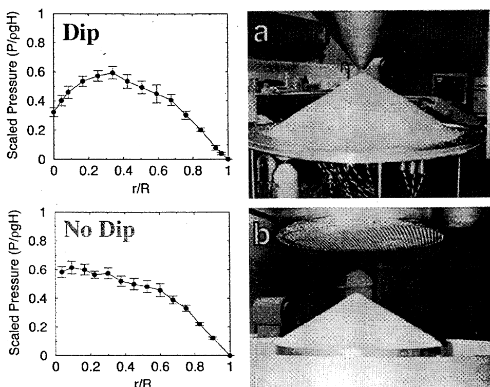
図 4: 砂山底部の垂直圧力分布. r は砂山の中心からの距離. H, R は, それぞれ砂山の高さと半径. (a) の砂山は一点から砂を落として作ったのに対して, (b) の砂山は円盤の上に様に砂を降り積もらせて作ったものである. それぞれの圧力分布を左側に示してある. (a) では中心で圧力分布にくぼみ (dip) があるのに対して, (b) にはくぼみはない. (Adapted from ref.[11])
