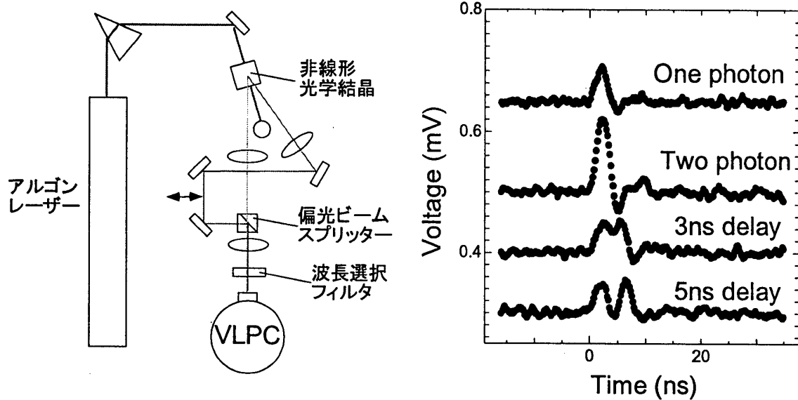
図6 光子数検出器
