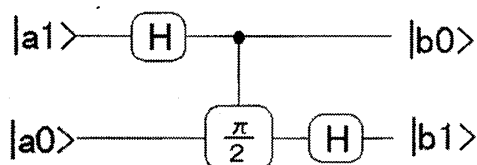
図9 量子フーリエ変換回路
