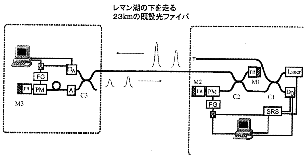
図5 量子暗号通信実験
