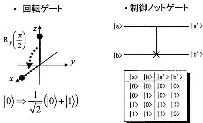
図8 基本量子ゲート
