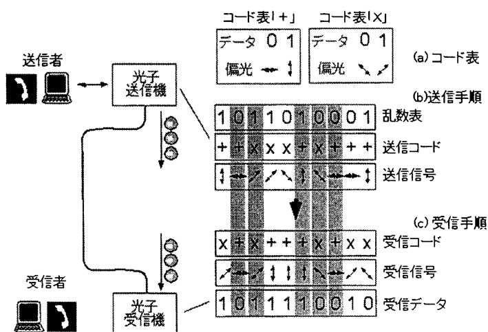
図4 量子暗号通信
