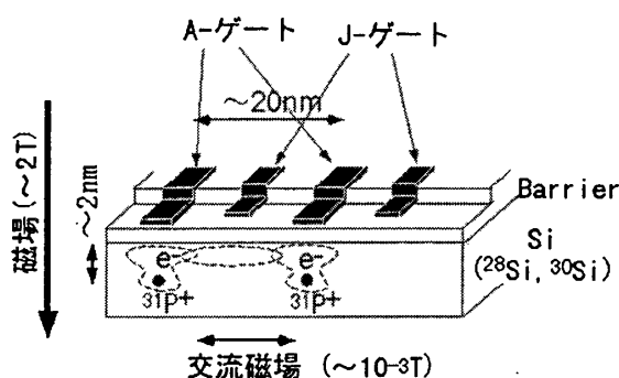
図11 シリコン量子計算機のアイデア
