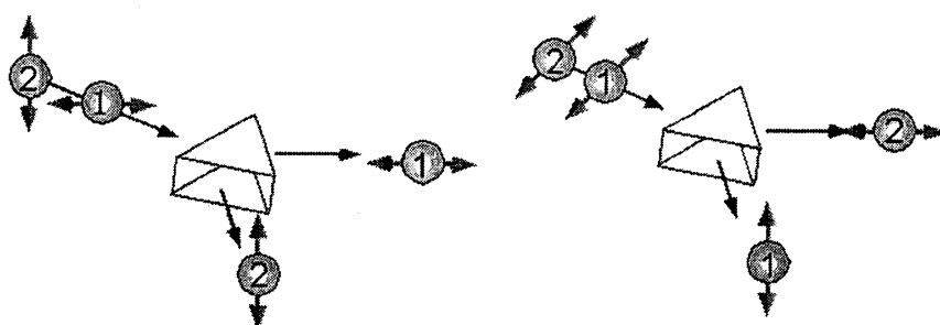
図3 光子の偏光
