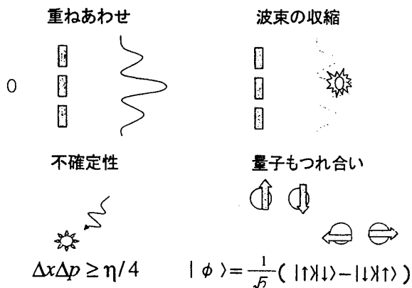
図1 量子力学の基本的な性質
