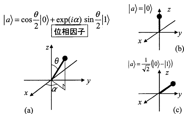
図7 量子ビット
