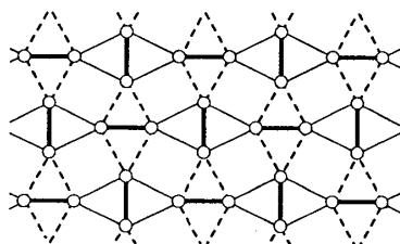
図1: 直交ダイマー模型。太線、細線、破線はそれぞれ反強磁性相互作用 J , J' , J'' を表している。太線のダイマーが直交しているので、直交ダイマー系と呼ばれている。
