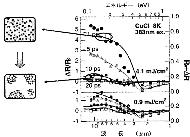
図 11 励起子共鳴 (383 nm) 励起下での、中赤外領域の過渡反射スペクトル (1, 5, 10, 20 ps)。励起光強度は (a) 4.1 (b) 0.9 mJ/cm 2 。実線は電子正孔液滴が生じて、部分的に電子正孔液滴を形成しイオン化している (左図) と仮定したときの反射スペクトルの計算値。[6]
