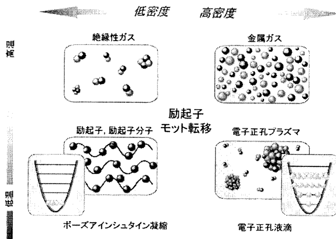
図 7 極低温高密度電子正孔系の諸相
