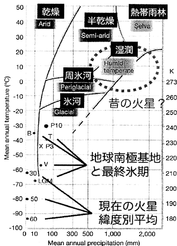
図 1: 気候が決める地形の種類 (Baker 2001 の図に追記) [1] 横軸 (年間降水量) 500 ミリ/年で降水・河川浸食優勢 (熱帯雨林・湿潤) と風浸食優勢 (乾燥・半乾燥) とが分かれる。また縦軸 (年平均気温) 氷点で周期的凍結破碎浸食もしくは氷河浸食優勢 (周氷河・氷河) とそれ以外とが分かれる。
