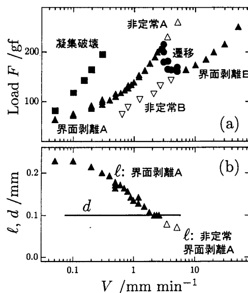
図5. (a) 引っ張り荷重と(b) d , \ell の速度依存性。白抜き記号は非定常遷移過程。温度@30°C
