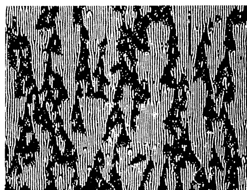
図4. 遷移域で粘着剤に残る時空パターン。剥離フロントは水平、下向きに進行。縞の間隔=100 \mu\text{m} 。
