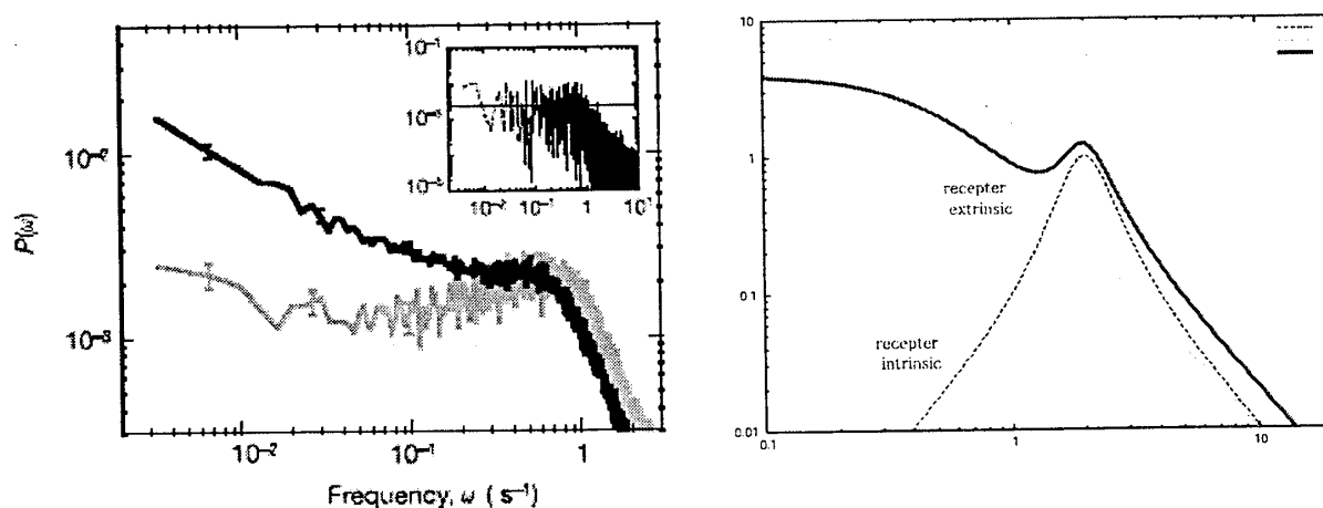
図4: (左図) 大腸菌のタンブリングの実測パワースペクトル (Cluzel. et. al.[4]より引用)。黒は野生型、灰はIPTG誘導によりCheR発現量を増やした変異型。変異型のほうが行動のパライティが下がる。(右図) 四状態モデルによるパワースペクトルの解釈。化学走性受容体由来のバンドパス型ゆらぎと他のローパス型ゆらぎの重ね合わせとして理解できる。
