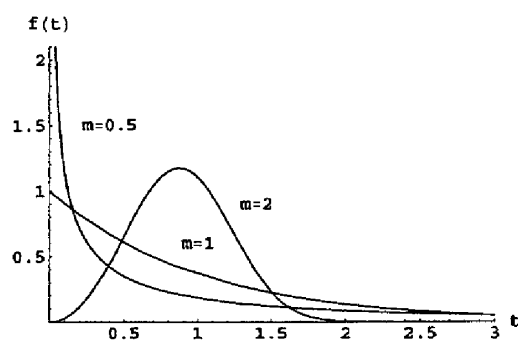
図 1: m の値の違いによる確率密度関数の形状 ( \alpha = 1 )
