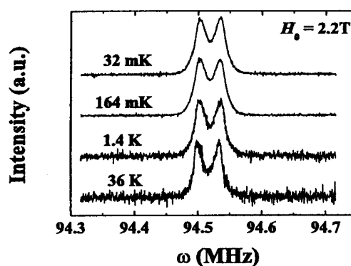
図 7: \kappa -(ET) 2 Cu 2 (CN) 3 塩の NMR スペクトルの温度依存性
