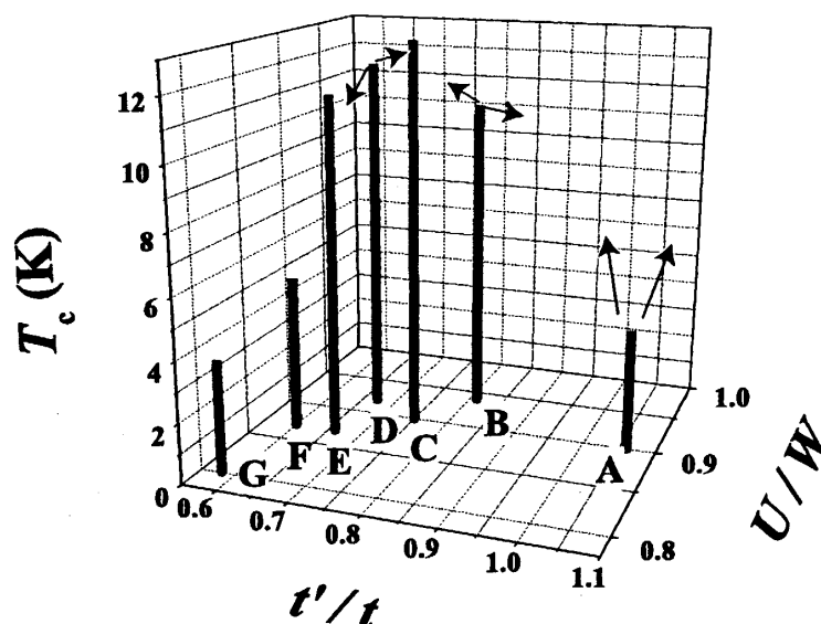
図 11: \kappa -(ET) _2 X 塩における T_C の t'/t および U/W 依存性。矢印は一軸性ひずみによる T_C の変化を示す。X = Cu _2 (CN) _3 (A), Cu(NCS) _2 (B), Cu[N(CN) _2 ]Cl (C), Cu[N(CN) _2 ]Br (D), Cu(CN)[N(CN) _2 ] (E), Ag(CN) _2 H _2 O (F), I _3 (G)。モット絶縁体 (A および C) の場合は、静水圧下での T_C を表示している
