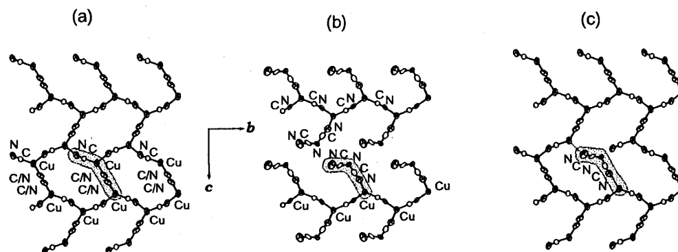
図 2: (a) \kappa\text{-(ET)}_2\text{Cu}_2(\text{CN})_3 の陰イオン層の構造、C/Nは炭素と窒素が無秩序（占有率 50 %）である事を示す。(b) \kappa\text{-(ET)}_2\text{Cu}(\text{CN})[\text{N}(\text{CN})_2] 塩の陰イオン層の構造、(c) \kappa' 塩の混合陰イオン層の構造の模式図。
