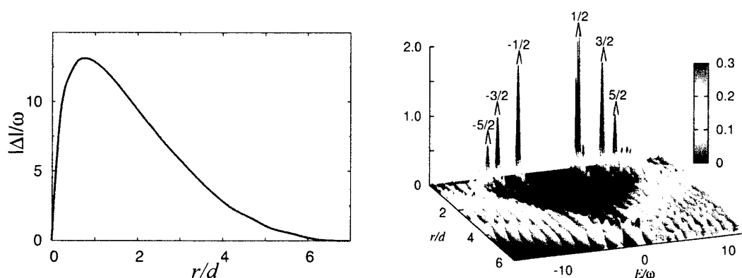
図 1: (左) 秩序パラメーター \Delta(\mathbf{r}) の空間依存性と (右) 局所状態密度 N(\mathbf{r}, E) \equiv N_{\uparrow}(\mathbf{r}, E) = N_{\downarrow}(\mathbf{r}, E) [式 (39, 40) 参照]. ここで d = \sqrt{\hbar/M\omega} , M は粒子質量, \omega はトラップポテンシャル周波数 (以下同様). 共に粒子数バランスの系. ただし, 動径方向に軸対称な調和振動子型のトラップポテンシャル V(r) \propto r^2 がある場合. (左) 秩序パラメーターに注目すると, 対ポテンシャルが量子渦中心から系の外側に向かって増加し, 井戸型ポテンシャルに似た形を持つことがわかる. これにより, 量子渦中心に離散的な状態ができる. (右) 局所状態密度中のラベルは角運動量 q_{\theta} を示す. これらのラベル付けされた状態を含むギャップ中の束縛状態は CdGM 状態と呼ばれる. q_{\theta} = 1/2 の振幅は非常に大きい, 図を見やすくするために上部を省いて描いている.
