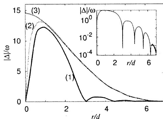
図 5: 秩序パラメーター \Delta(r) の空間変化. g = -1.5 . (1) は粒子数インバランス P = 0.3 で量子渦がある場合. (2) [(3)] は粒子数が等しく量子渦がある [無い] 場合. 挿入図は (1) の対数プロット.
