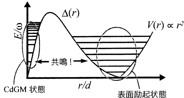
図 12: 対ポテンシャルとトラップポテンシャルによりできる、離散的な CdGM 状態と表面励起状態の概念図
