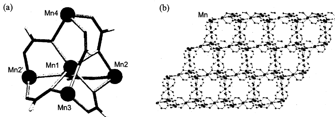
図 7 多孔性フェリ磁性体 [\text{Mn}_3(\text{HCOO})_6] : 蟻酸架橋による (a) \text{Mn}^{\text{II}} 5核ユニットと(b) 一次元チャンネル型細孔を有する骨格構造
