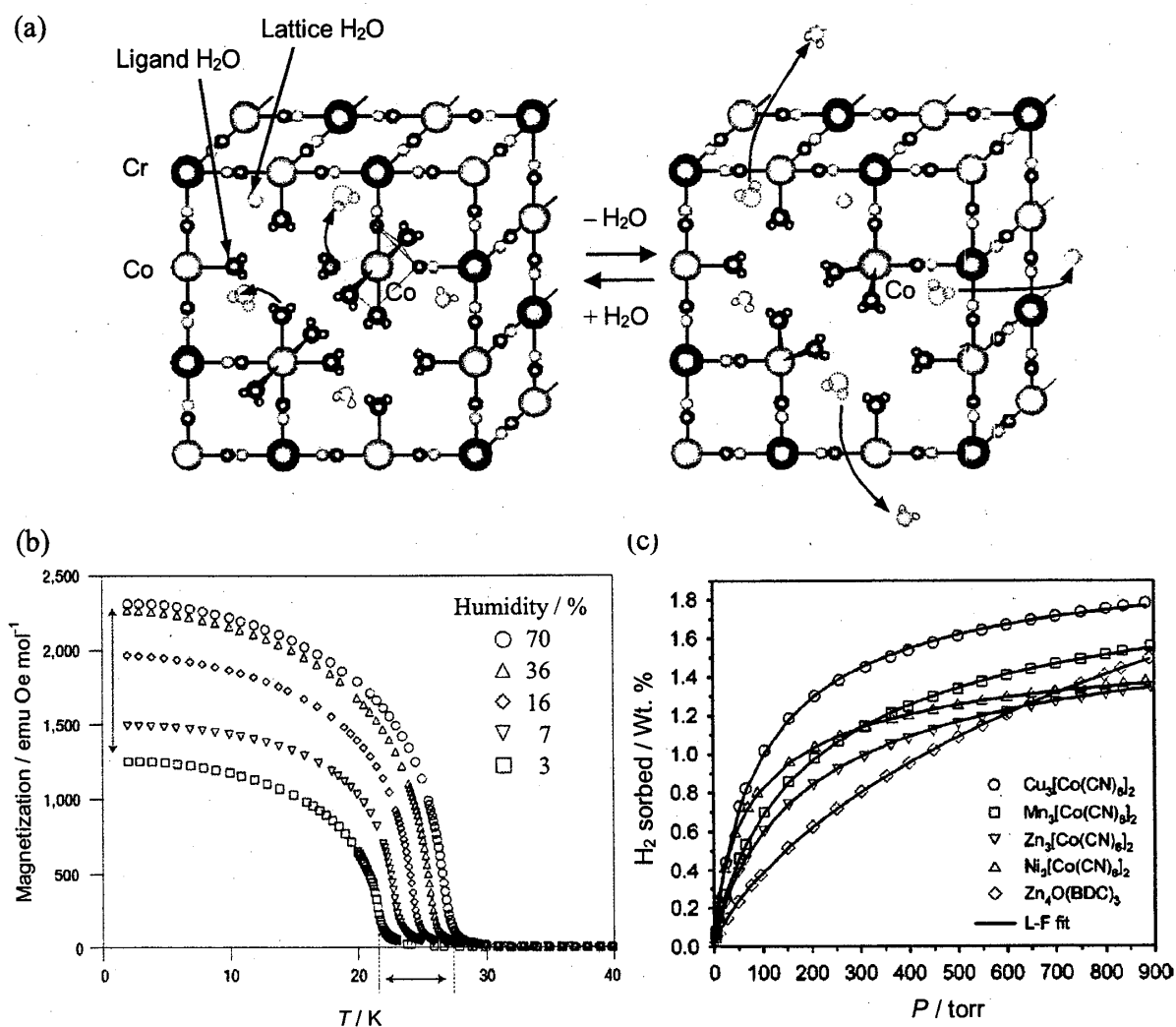
図 6 Prussian-blue 類縁体 \text{Co}^{\text{II}}[\text{Cr}^{\text{III}}(\text{CN})_6]_{2/3} \cdot z\text{H}_2\text{O} の (a) 脱水による構造変化の模式図、(b) 磁気挙動の湿度依存性、(c) \text{M}^{\text{II}}_3[\text{Co}^{\text{III}}(\text{CN})_6]_2 ( \text{M} = \text{Cu}, \text{Mn}, \text{Zn}, \text{Ni} ) の水素吸着能
