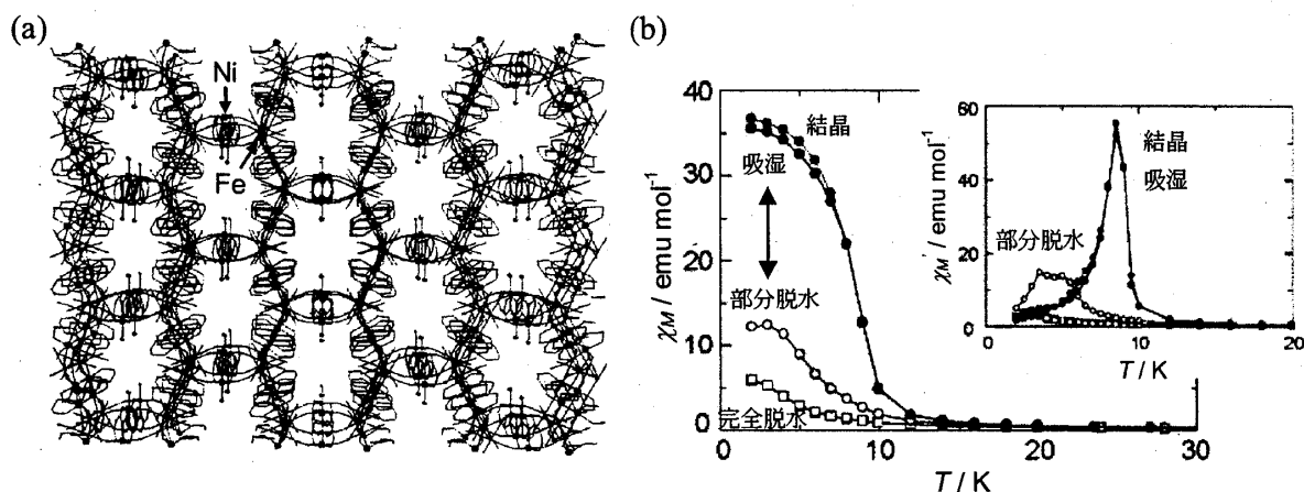
図 3 三次元 \text{Ni}^{\text{II}}/\text{Fe}^{\text{III}} 強磁性体 [\text{Ni}(\text{dipn})]_2[\text{Ni}(\text{dipn})(\text{H}_2\text{O})][\text{Fe}(\text{CN})_6]_2 \cdot \text{H}_2\text{O} : (a) Honeycomb 型チャンネル構造、(b) 水の吸脱着による直流及び交流磁気挙動の可逆的变化
