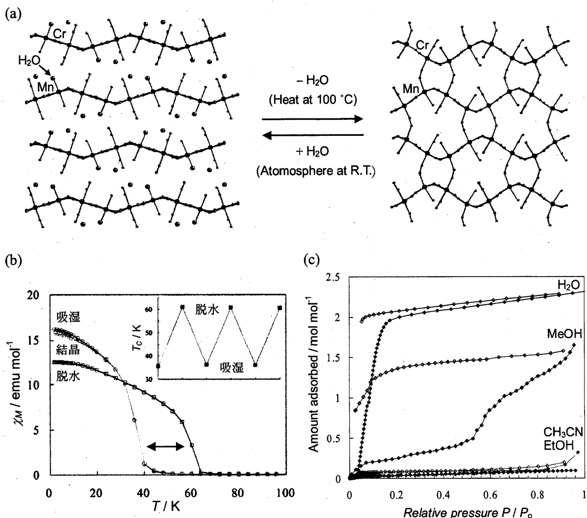
図 5 二次元 \text{Mn}^{\text{II}}\text{Cr}^{\text{III}} フェリ磁性体 [\text{Mn}(\text{NNdmenH})(\text{H}_2\text{O})][\text{Cr}(\text{CN})_6] \cdot \text{H}_2\text{O} : 配位水の吸脱着による (a) 二次元及び三次元構造間の変換と (b) 磁気特性の変化、(c) 脱水相の室温における溶媒の吸着等温線
