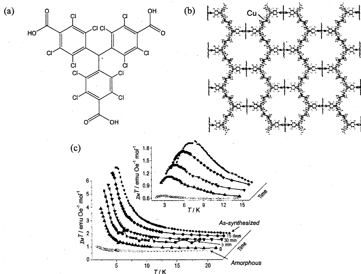
図 1 (a) 常磁性有機ラジカル架橋配位子 H 3 PTMTC、(b) MOROF-1 の二次元シート構造、(c) 合成直後と水の脱水及び再吸着による磁気挙動の変化
