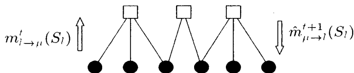
図 19: BP におけるグラフの伝播
