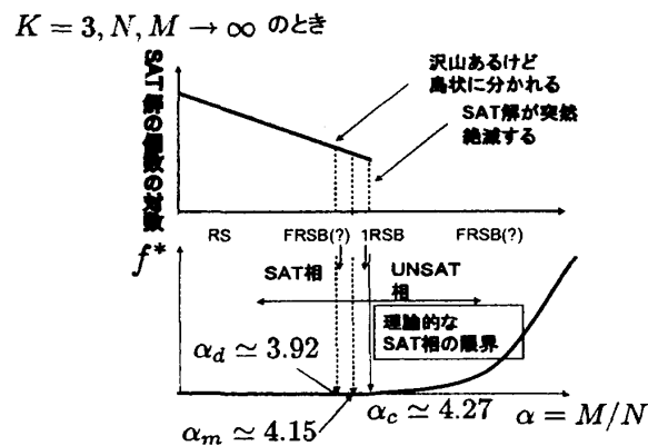
図 4: SAT 問題についてレプリカ解析から得られる描像
