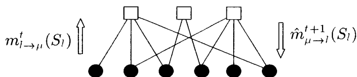
図 22: Loopy BP
