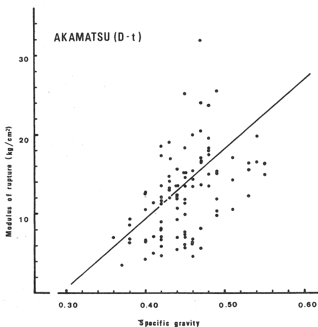
Fig. 6 アカマツ (D) 曲げ強さ (よこ) と比重 Modulus of rupture of Akamatsu (D) versus specific gravity (transverse).
