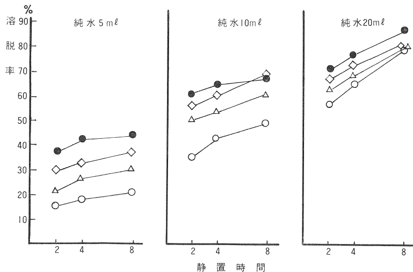
図 3. 静置状態における溶脱率
