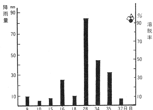
埋め込み日より回収日までの降雨経過 注：記号は図3と同じ
