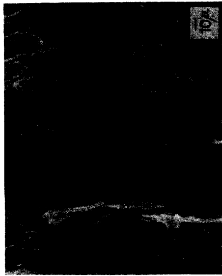
(g) フェノール樹脂注入処理材 (イタヤカエデ 放射断面)
