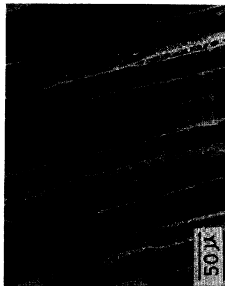
(d) エポキシ樹脂注入処理材 (ヒノキ 心材 放射断面)
