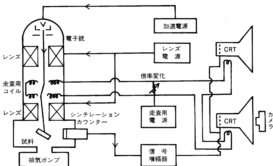
図2. SEMの原理図
