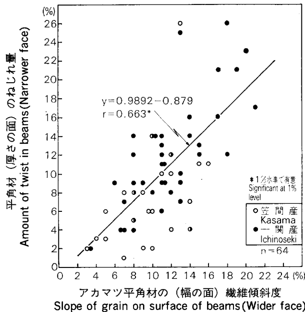
Fig. 8. 平角材の繊維傾斜度とねじれ量との関係
