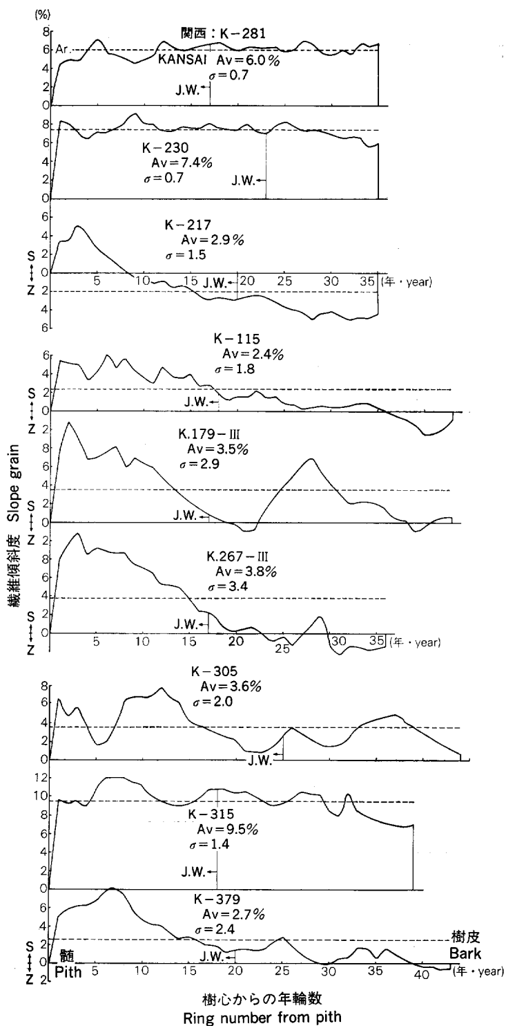
Fig. 2. 繊維傾斜度の樹心から外側までの各年の変化 (関西)
