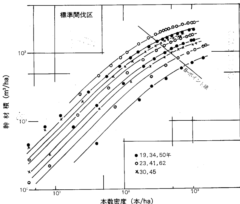
図7. 試験区別Y—N曲線
