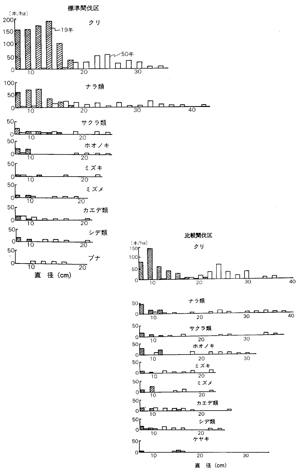
図4. 有用樹種別の直径分布
