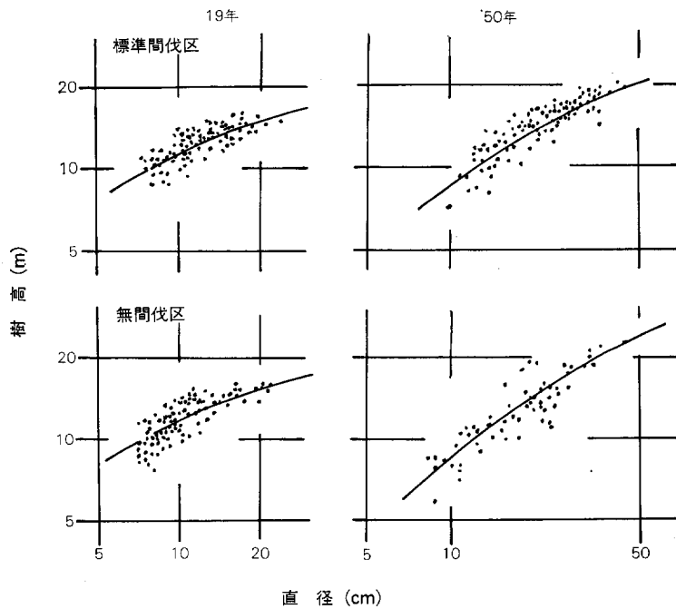
図5. D-H 曲線
