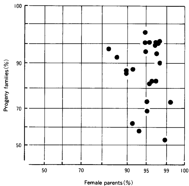
Fig.5. 充実率における母樹と子供家系の関係
