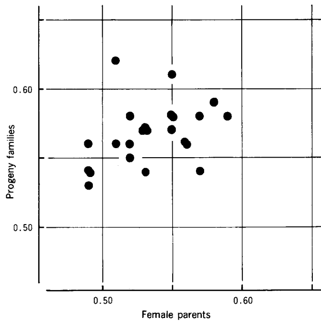
Fig. 3. 球果形状比における母樹と子供家系の関係
