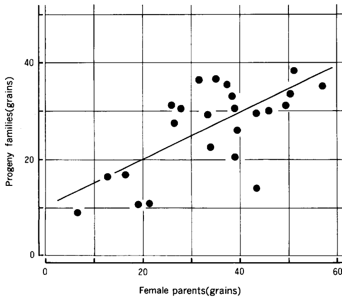
Fig. 4. 球果あたりの種子数における母樹と子供家系の関係
