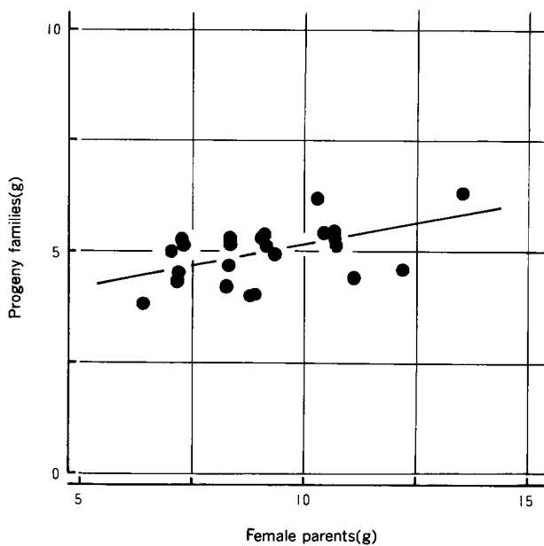
Fig.6. 1000 粒重における母樹と子供家系の関係
