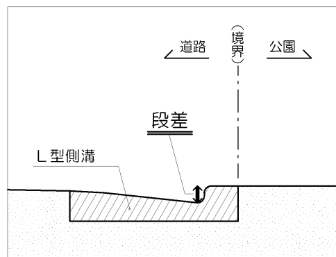
L型側溝の断面（概略図）
