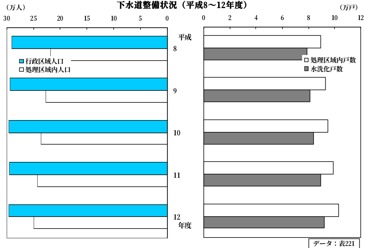
下水道整備状況（平成8～12年度）
