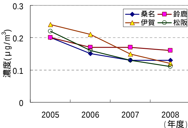
図4 クロロホルムの経年変化
