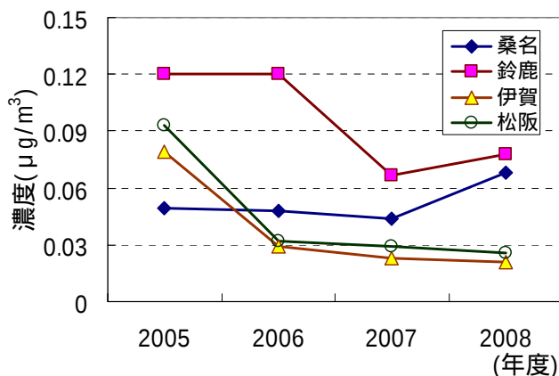
図2 アクリロニトリルの経年変化
