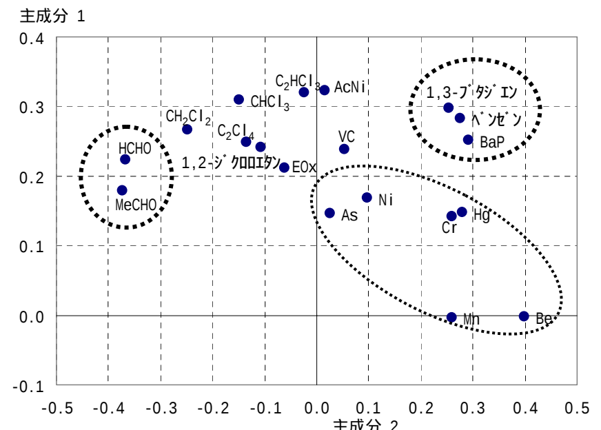
図 26 鈴鹿 固有ベクトルの散布図
