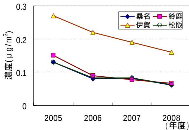
図 7 テトラクロロエチレン経年変化
