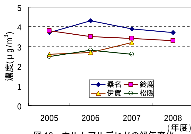
図 13 ホルムアルデヒドの経年変化
