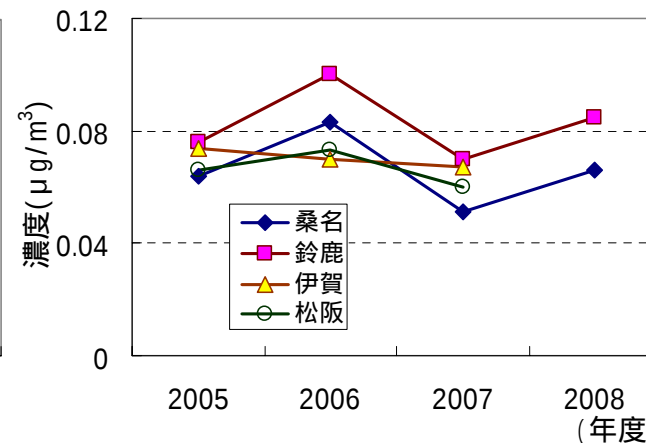
図 11 酸化エチレンの経年変化
