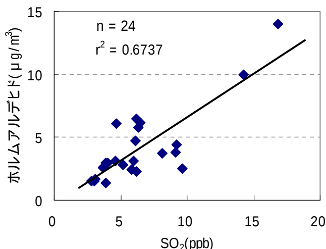
図23 桑名でのSO 2 とホルムアルデヒドとの関係 (2006～2007年度)
