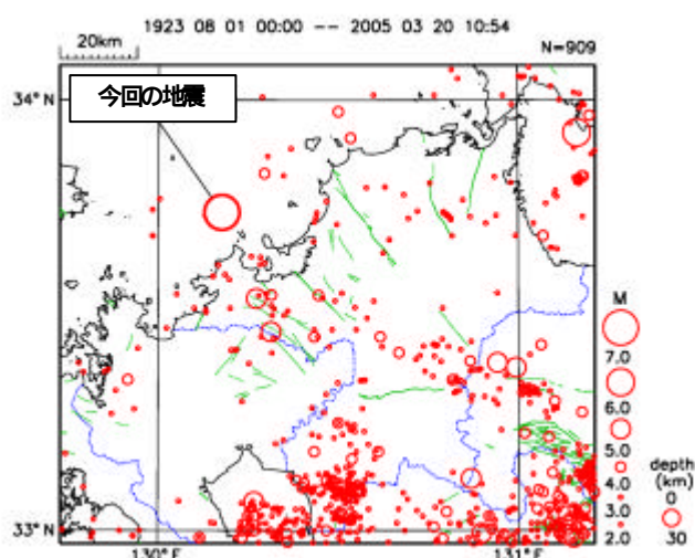
図7 震央分布図
