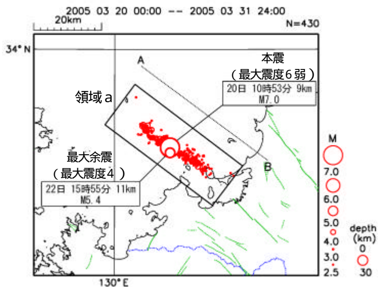
図3 震央分布図 (M 2.5、深さ 30 km)
