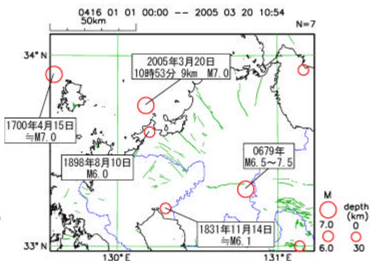
図8 震央分布図
