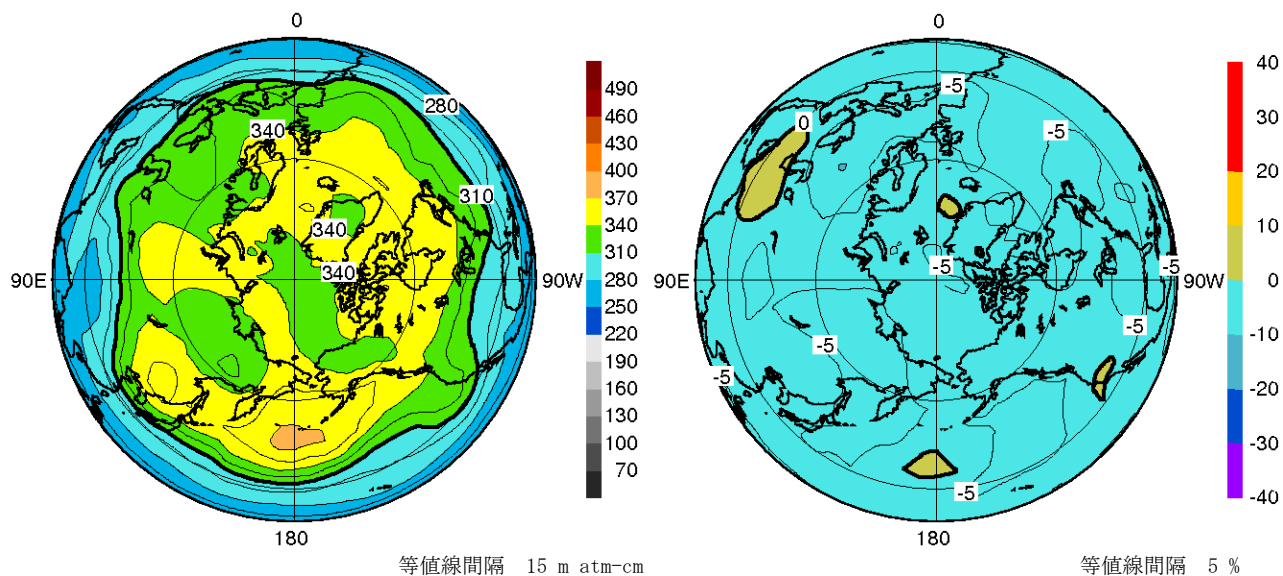
図 14 北半球の月平均オゾン全量（左）と参照値からの偏差（右）（2009 年 6 月）
