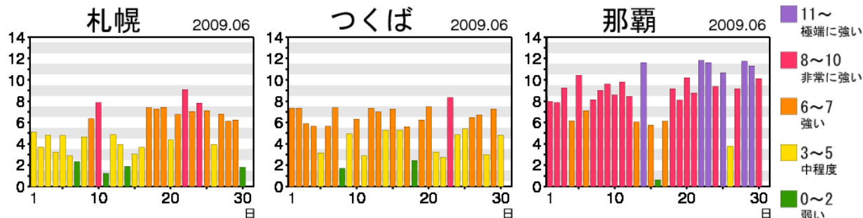
図4 日最大UVインデックスの推移（2009年6月）
