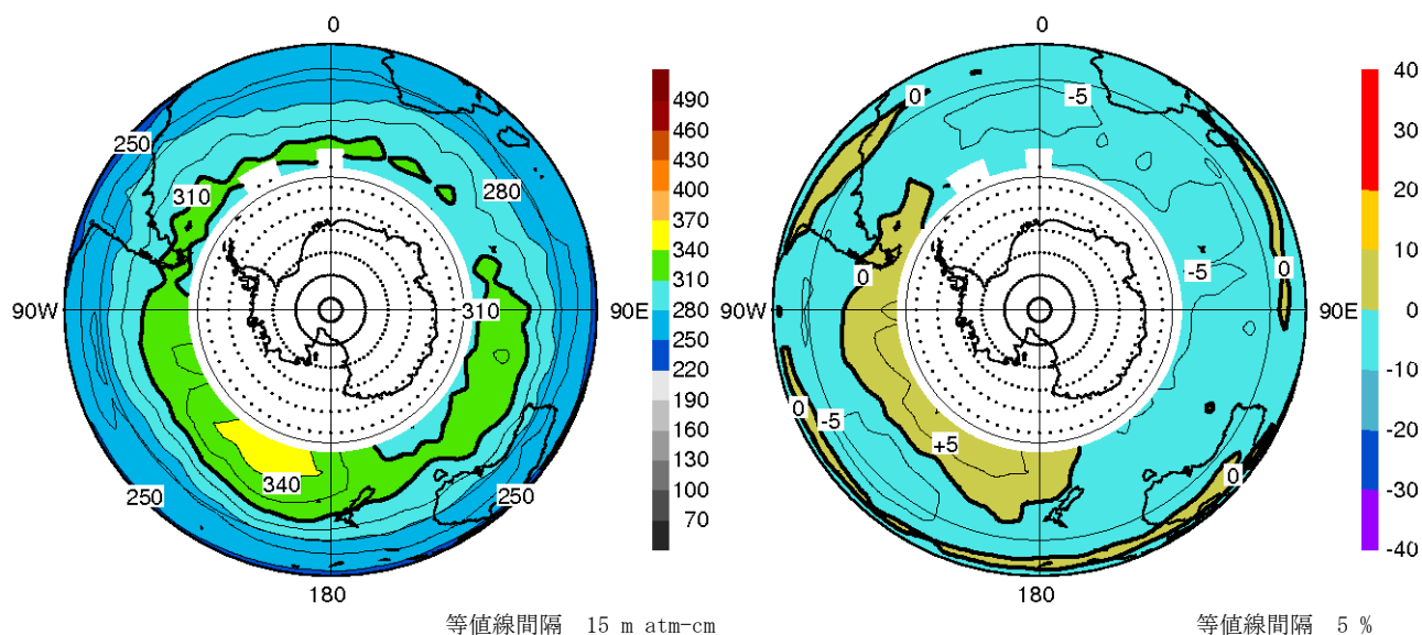
図 15 南半球の月平均オゾン全量（左）と参照値からの偏差（右）（2009 年 6 月）
