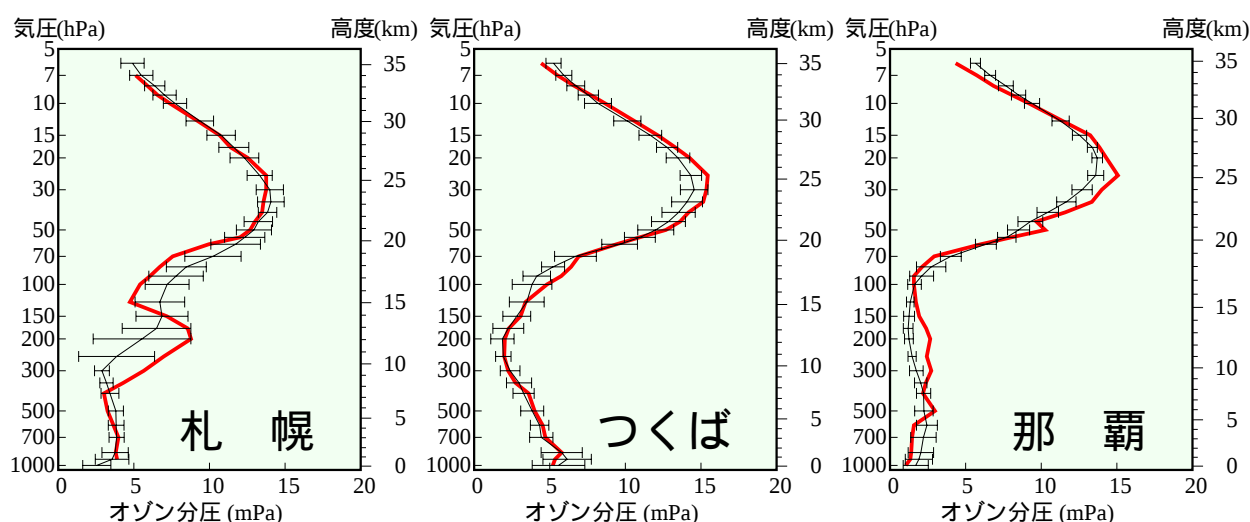
図2 オゾン分圧の高度分布（2009年6月）
