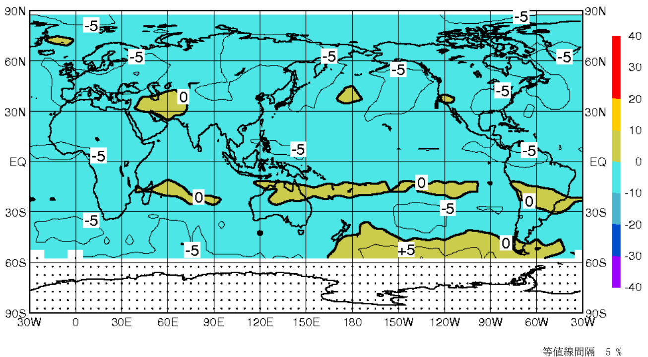
図 13 月平均オゾン全量の参照値からの偏差（2009 年 6 月）
