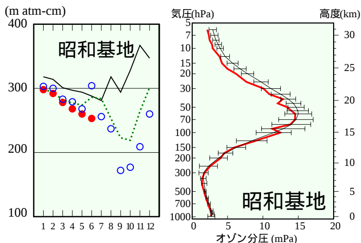
図8 (左) オゾン全量の月平均値の推移
