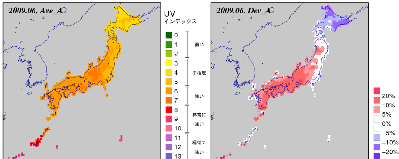
図5 日最大 UV インデックス（解析値）の月平均値（左）と参照値からの偏差（右）（2009年6月）
