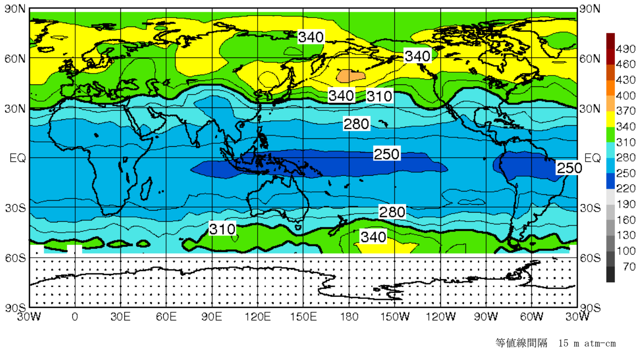
図 12 月平均オゾン全量（2009 年 6 月）
