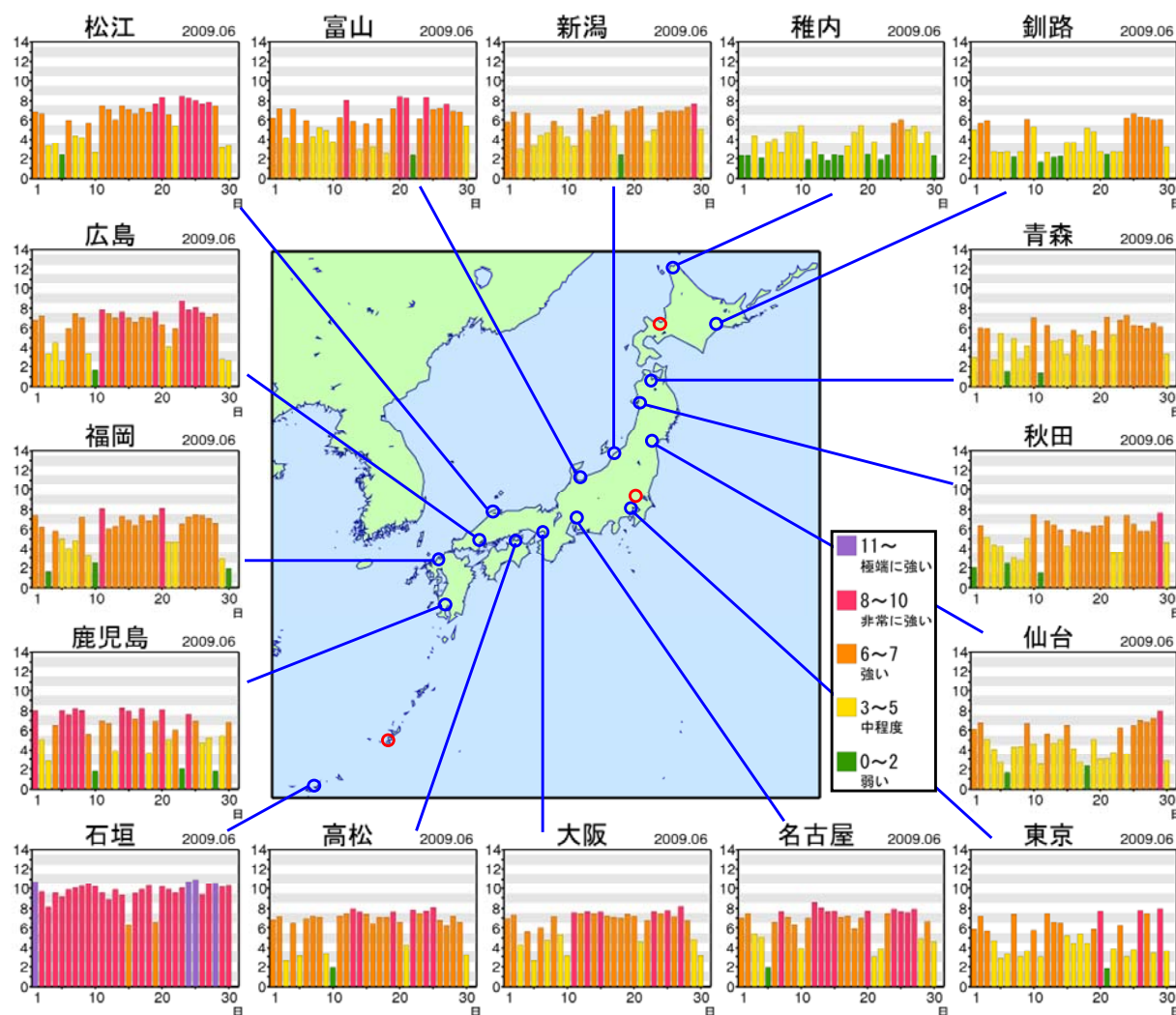
図6 日最大 UV インデックス（解析値）の推移（2009年6月）
