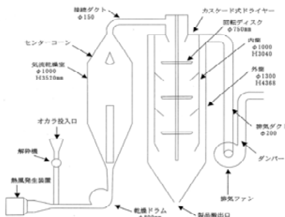
図1 カスケード式乾燥試験装置
